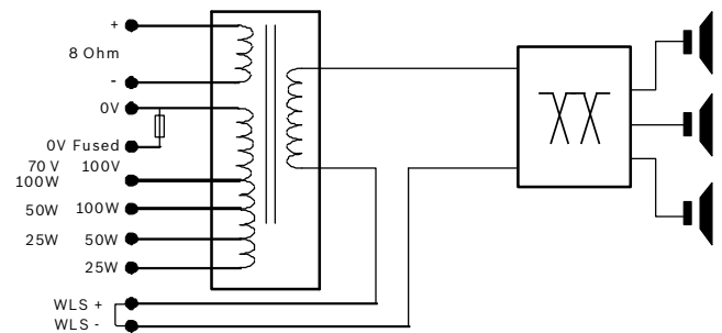
Schemat połączeń
