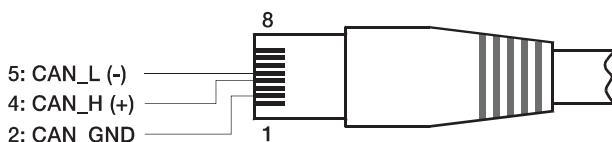
Rysunek 6.8: Schemat złącza CAN
