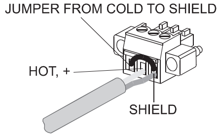
Rysunek 6.2: Kable niesymetryczne
