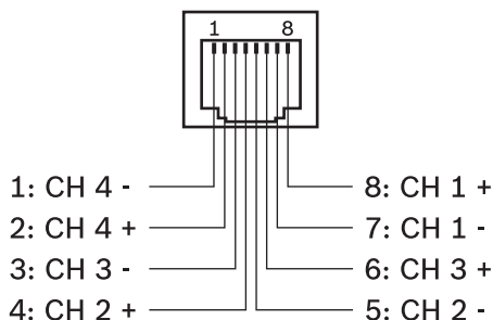
Rysunek 6.4: Przyporządkowanie styków gniazda LINE OUT 1-4
