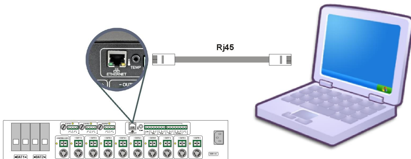
Rys. 23. Schemat połączenia zasilacza z komputerem.
