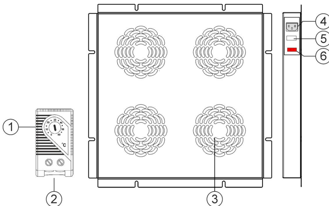
Rys. 13. Panel wentylatorów z termostatem.
