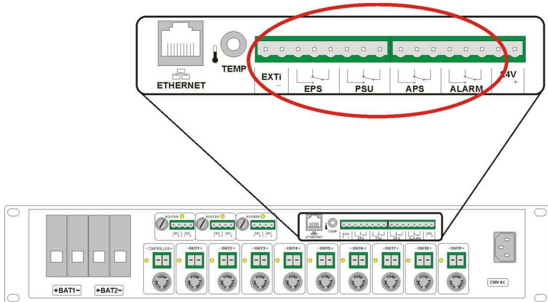
Rys. 20. Wyjścia/wejścia techniczne zasilacza.
