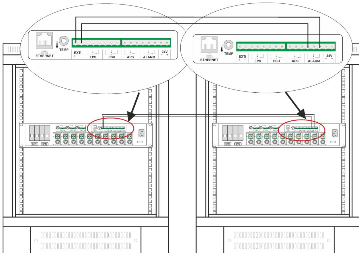
Rys. 21. Schemat poglądowy podłączenia sygnału awarii zbiorczej.
