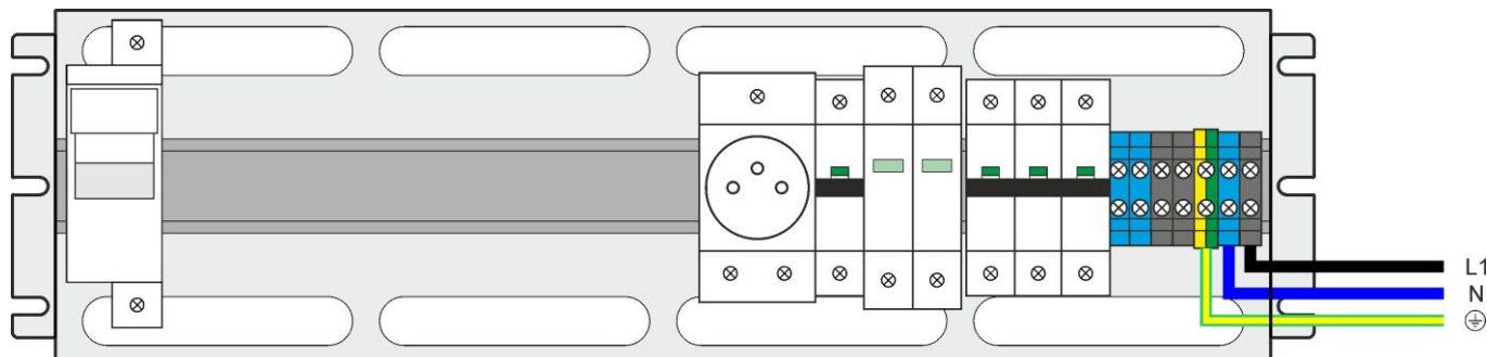
Rys. 44. Podłączenie do instalacji elektroenergetycznej – przyłączy 1 fazowe 230V AC.
