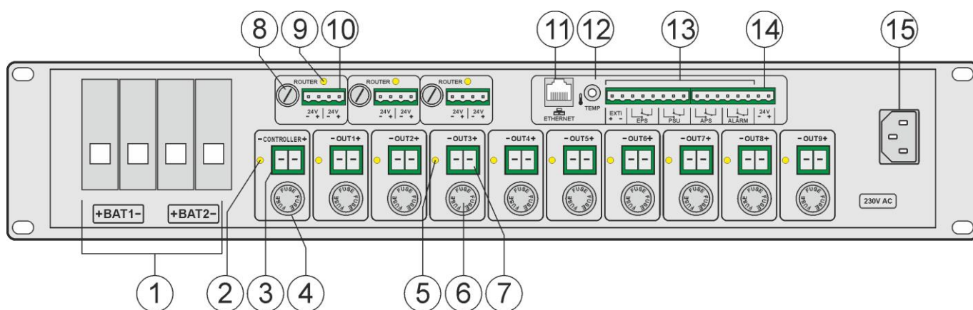
Rys. 16. Panel tylny zasilacza w wersji konfiguracji maksymalnej.
