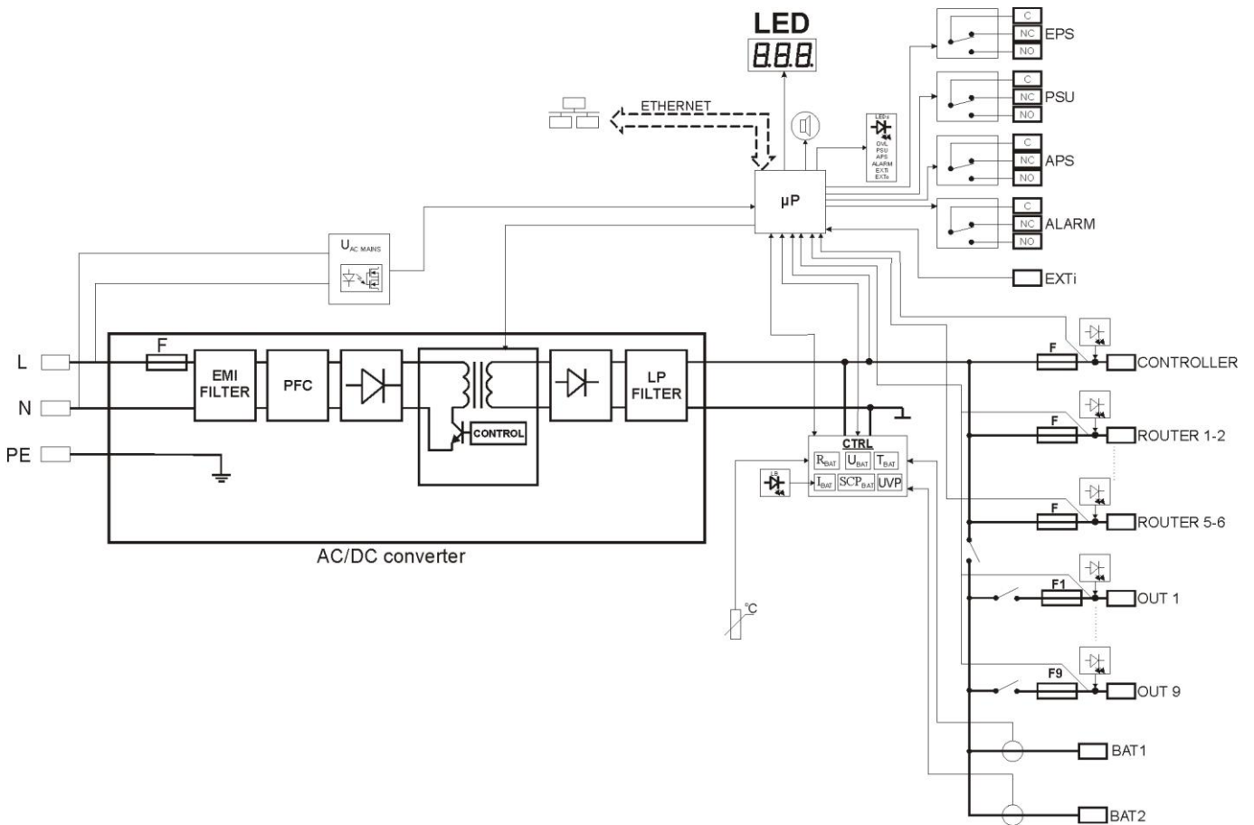
Rys. 14. Schemat blokowy zasilacza.
