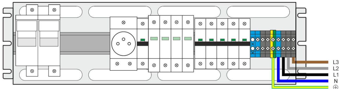
Rys.45. Podłączenie do instalacji elektroenergetycznej – przyłącze 3 fazowe 230/400V AC.
