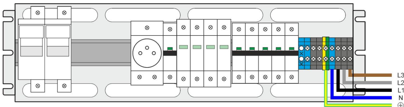
Rys.8. Podłączenie do instalacji elektroenergetycznej – przyłącze 3 fazowe 400V AC.
