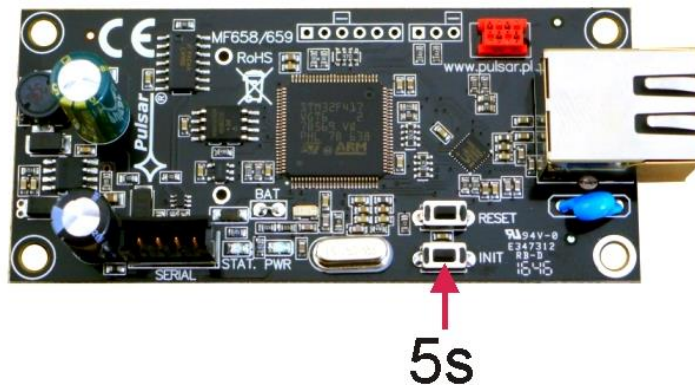
Rys. 26. Widok modułu Ethernet
